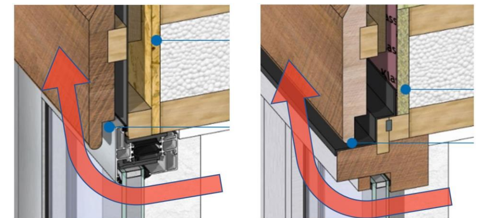
figuur 12. De oriëntatie van ventilatiespleten heeft veel invloed op de kans dat uitslaande vlammen snel de spouw in slaan.
