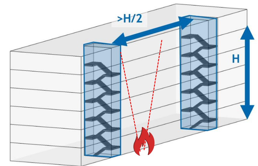
figuur 6. Ligging vluchtroutes. De rode stippellijnen geven de grenzen van het initiële brandvoortplantingsgebied over de gevel bij de aangegeven brandpositie.
