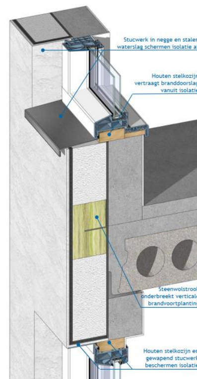
figuur 9. Een onderbreking van de isolatie met een steenwolstrook.
