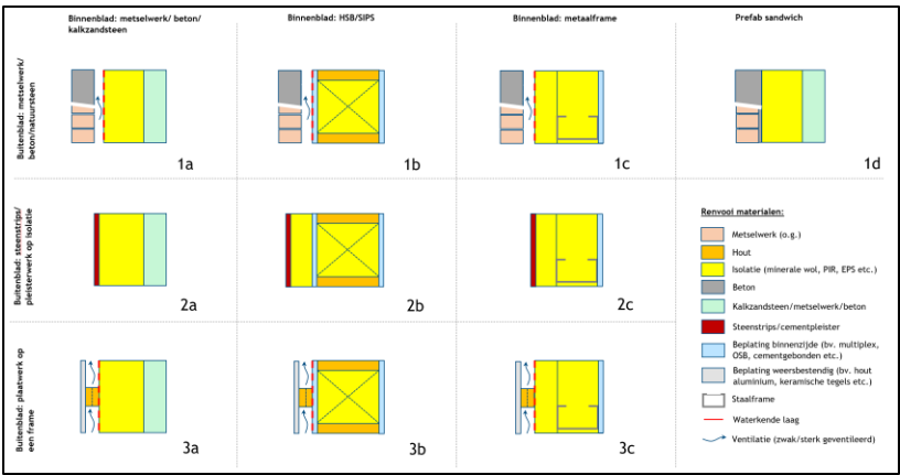
figuur 5. De onderscheiden geveltypen (zie ook bijlage 3)
