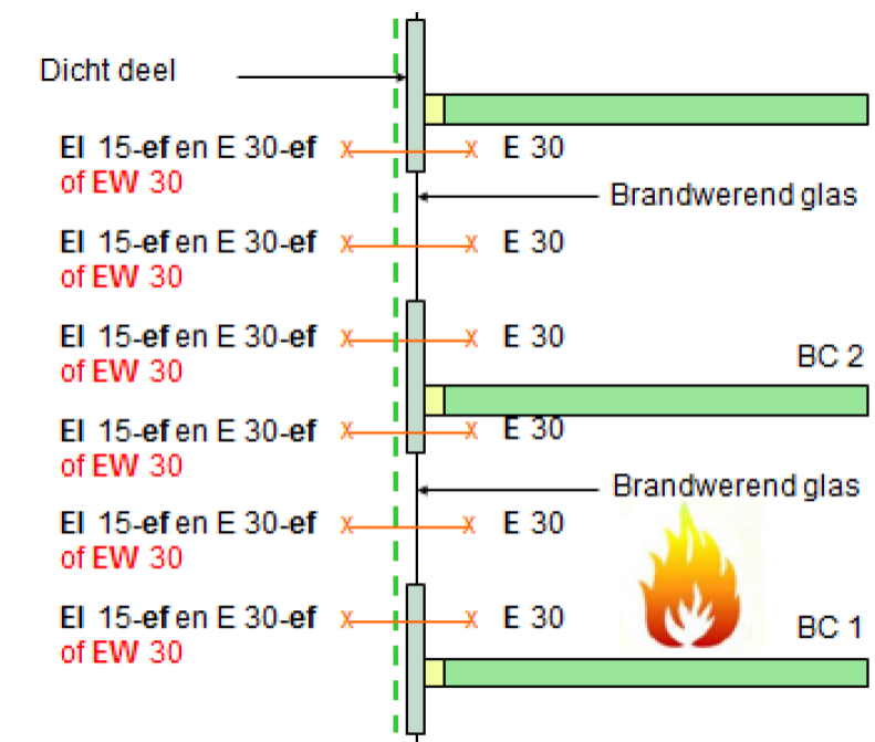
figuur 11. Voorbeeld van brandwerendheidscriteria voor geveldelen uit NEN 6069:2019
